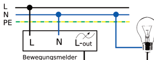
Anschlussbild 3-Draht Bewegungsmelder
