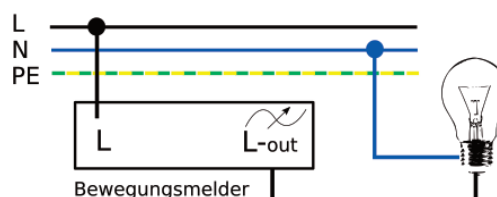
Anschlussbild 2-Draht Bewegungsmelder
