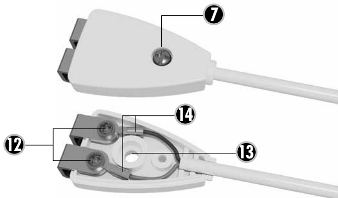
ABB. 2 WASSER-SENSOR
