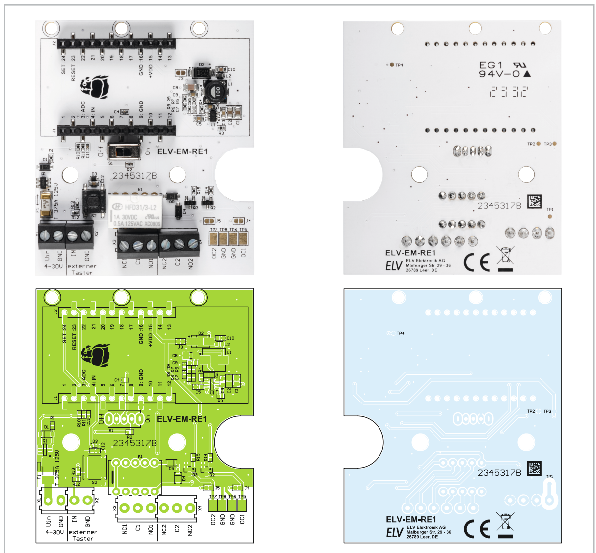
Bild 5: Platinenfotos und Bestückungsdrucke des ELV-EM-RE1
