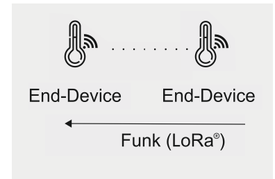
Bild 2: Architektur der LoRa®-Funkstrecke
