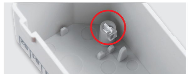
Bild 18: So erfolgt das Einsetzen des Lichtleiters in das Gehäuseoberteil.
