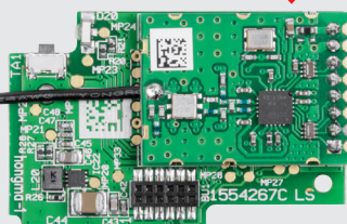
Bild 7: Platinenfotos der vollständig bestückten Controllereinheit mit zugehörigen Bestückungsplänen, oben ohne TRX-Modul, unten mit TRX-Modul
