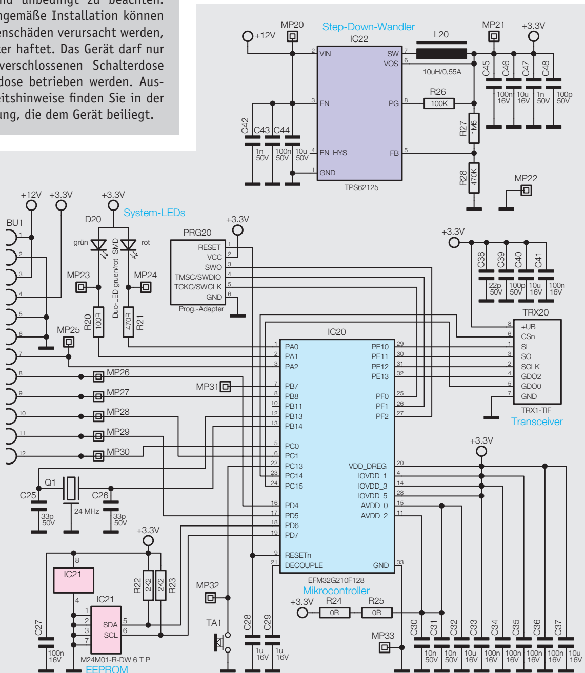
Bild 5: Das Schaltbild der Controllerplatine der Aktoren
