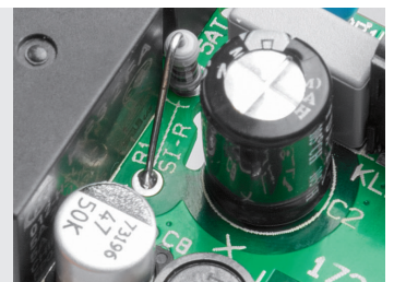
Bild 8: So ist der Sicherungswiderstand R1 einzubauen.
